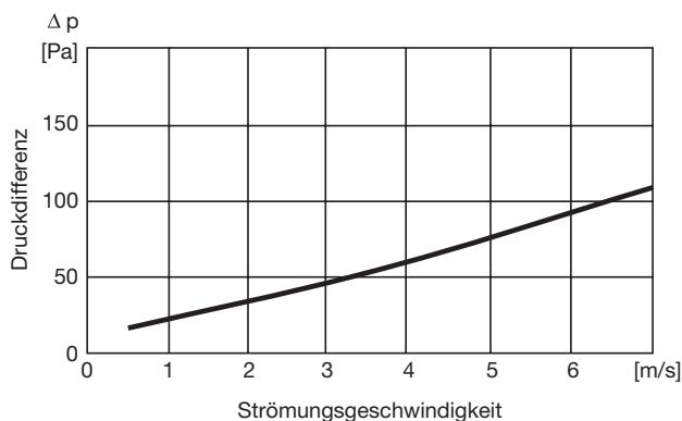
Widerstandskennlinie für G4 Filter
